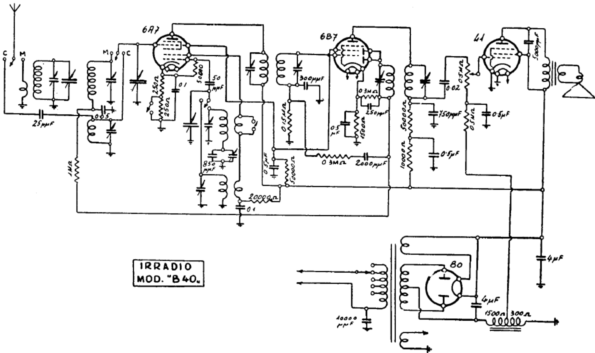
IRRADIO — Modello « B 40 ». - Produzione: 1935. - Media frequenza: 250 kc.
